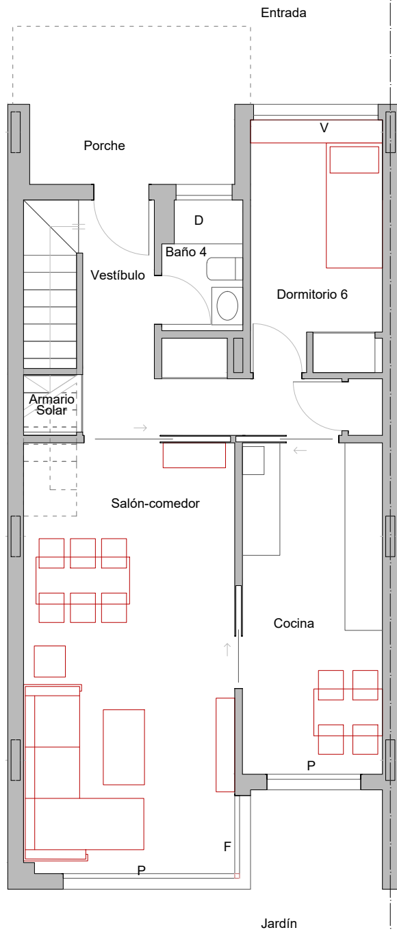
Planta baja
